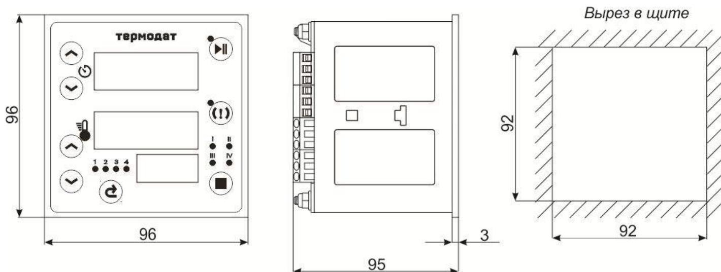
Рисунок 8 – Габаритные размеры прибора Термодат-12Т6/...и 12Т6-А...
