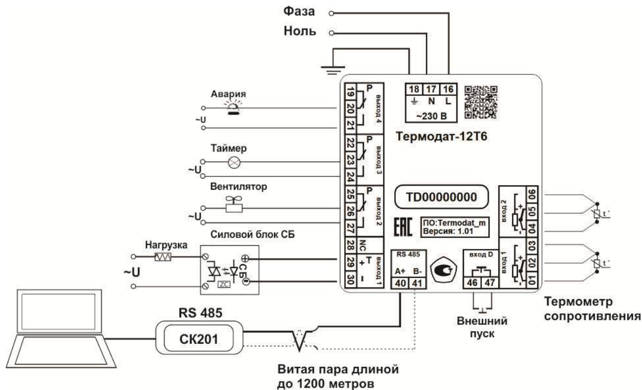
Рисунок 7 – Схема подключения прибора.
