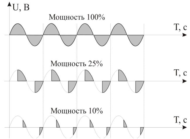
Рисунок 1. Фазоимпульсное управление
