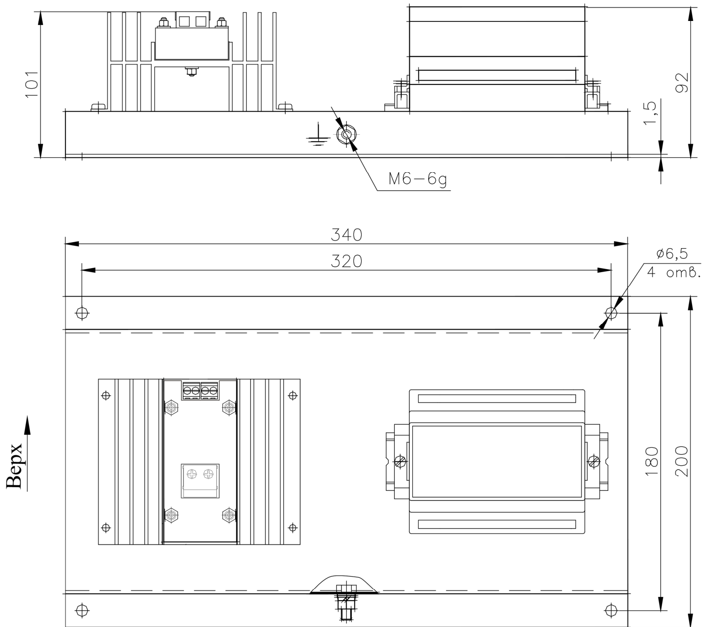
Рисунок 2. Габаритно-установочные размеры
